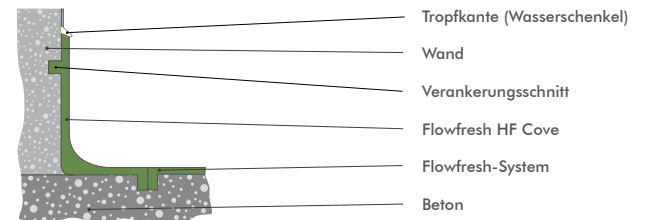
Typisches Detail für Boden-zu-Wand-Übergang
