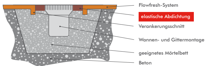
Typische Anordnung für Entwässerungsrinne
